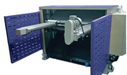
▶ Back Gauge
